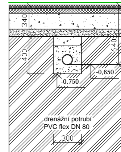
DETAIL PLOŠNÉ DRENÁŽE začátek M 1:25
