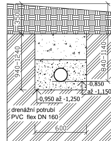
DETAIL SBĚRNÉ DRENÁŽE M 1:25
