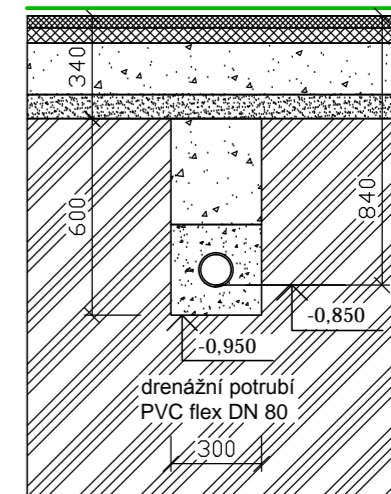
DETAIL PLOŠNÉ DRENÁŽE konec M 1:25
